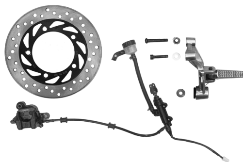
盘式制动器的结构图
