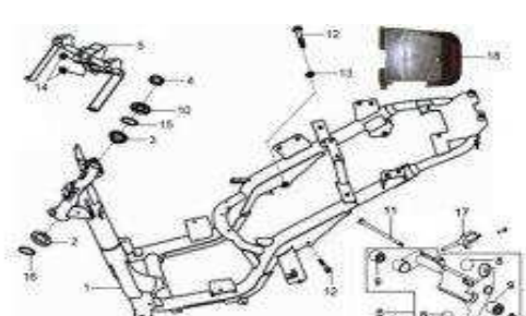
F11 FRAME BODY
