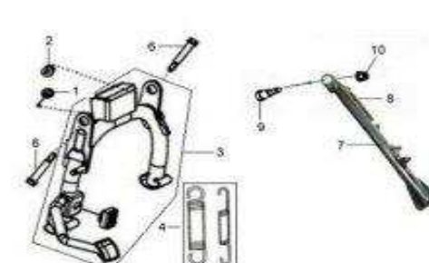
F12 MAIN STAND
