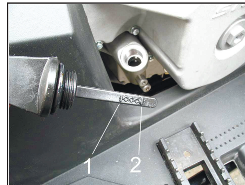
1. Максимальный уровень 2. Минимальный уровень
