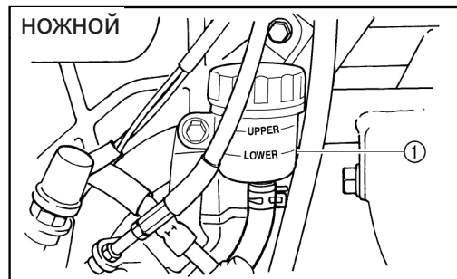
1. Минимальный уровень тормозной жидкости.
