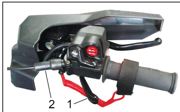
1. Рычаг газа 2. Тросик газа
