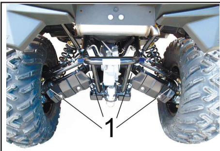
1. Пыльники задней оси (по 2 шт. на каждую сторону).
