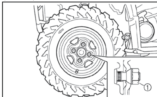
1. Колесная коническая гайка (4 шт.).
