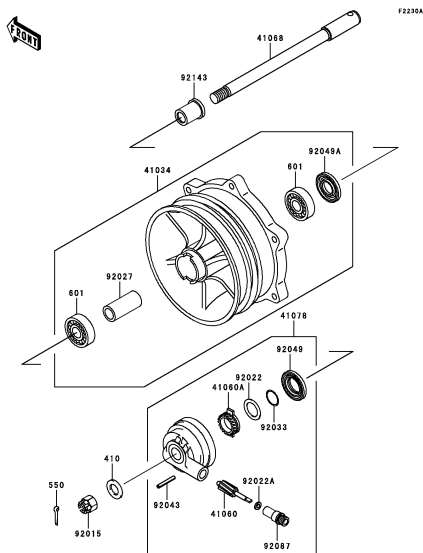
E-3 Front Hub(M6F)
