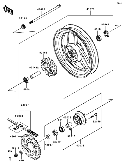
E-4 Rear Hub(L6F)
