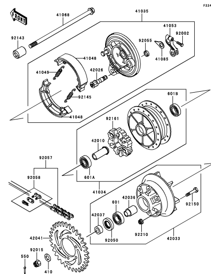
E-5 Rear Hub(M6F)
