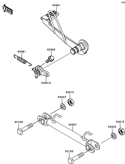
E-6 Brake Pedal(L6F)
