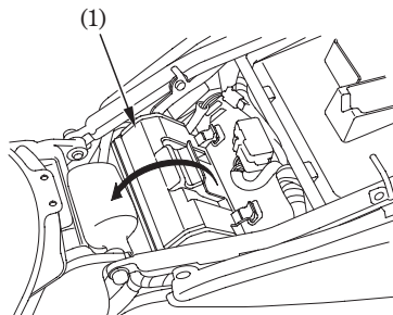
(1) Tapa de la caja de la batería
