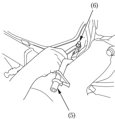
(5) Capuchón de la bujía (6) Llave de bujías
