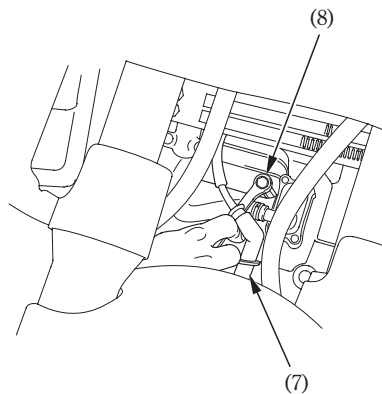
(7) Capuchón de la bujía (8) Llave de bujías
