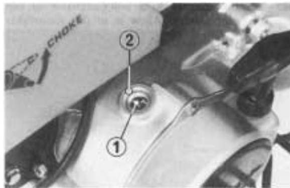
(1) T mark
