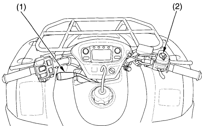
(1) shift lever
