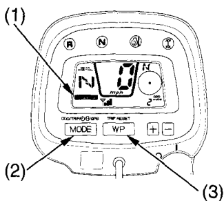
TRX400FGA
