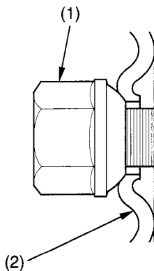
(2) wheel rim
