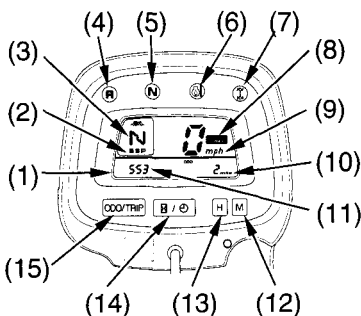
TRX400FA
