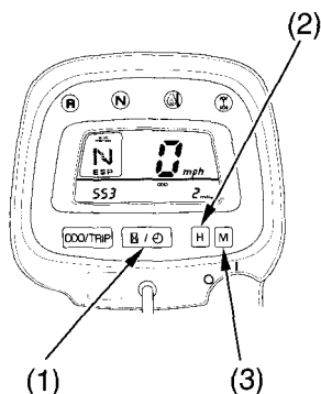
TRX400FA
