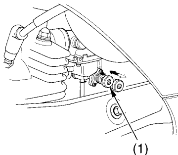
(1) starting primer knob
