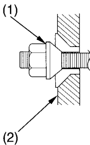
(2) wheel rim
