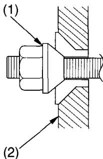
(2) wheel rim
