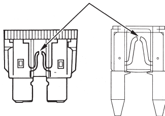
Fusible fundido
