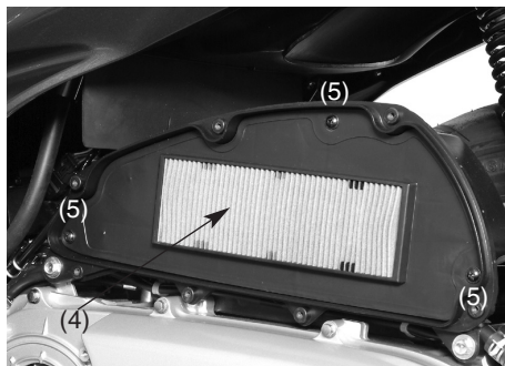
(4) Filtro de aire (5) Tornillos internos
