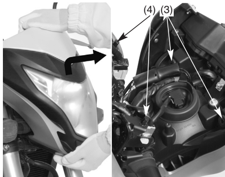
(3) Casquillo faro (4) Tornillos bastidor
