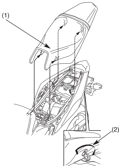
(1) Asiento
