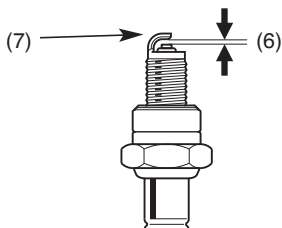
(6) Separación entre electrodos (7) Electrodo lateral
