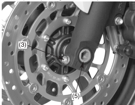
(3) Bulone de apriete del eje de la rueda (5) Eje delantero
