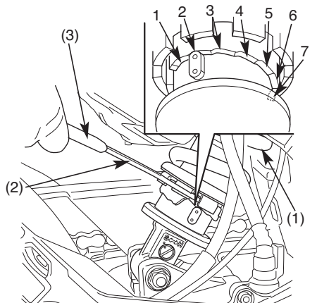
(1) Amortiguador (2) Llave de gancho
