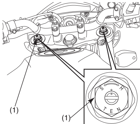
(1) Regulación precarga
