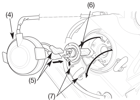
(4) Guardapolvos (5) Casquillo
