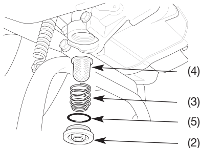
(2) Tapón de drenaje del aceite
