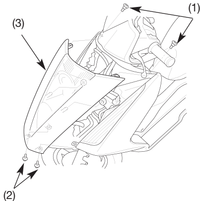
(1) Tornillos A (2) Tornillos B
