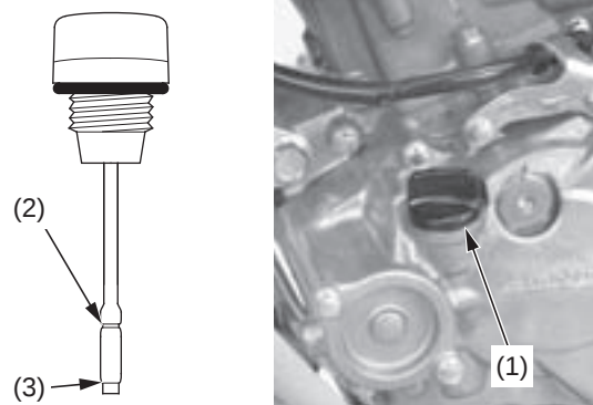
(1) tapa de relleno/varilla de medición del nivel de aceite de motor (2) marca de nivel superior (3) marca de nivel inferior
