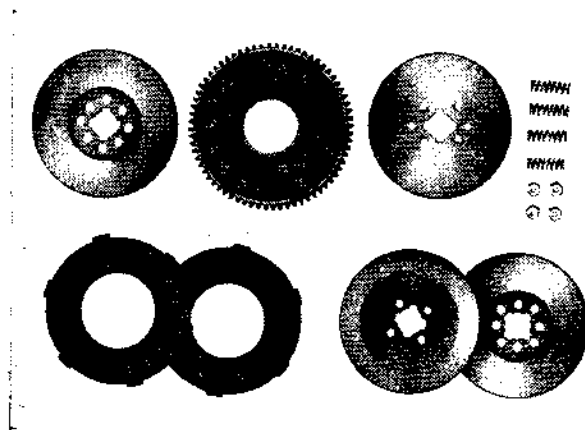
Abb. 18. Kupplung in Einzelteile zerlegt: Oben in der Mitte die zentrale Antriebsscheibe, links darunter die beiden Belagslamellen (Kork bzw. Jurid), daneben die entsprechenden Stahlscheiben. Die gesamte Kupplung arbeitet im Ölbad.
