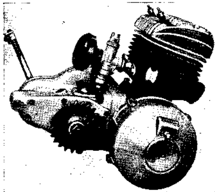
Abb. 4. Motor- getriebeblock des Typ SB500 (Licht- maschinen- u. Anlasserseite)
