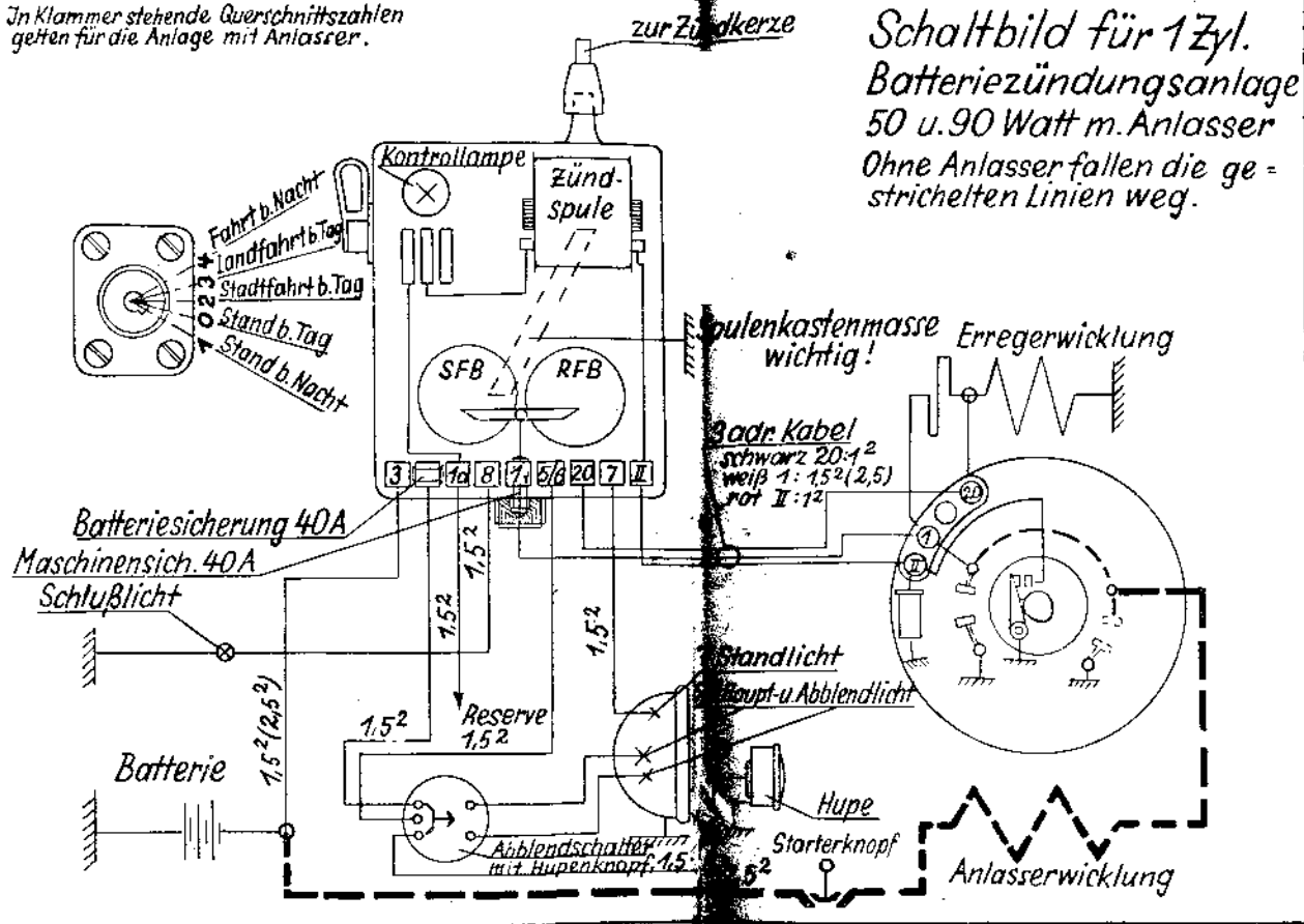
Abb. 51. Elektrisches Schaltbild für 1-Zylinder-Anlagen.
