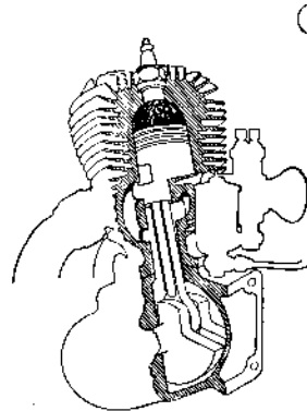
Abb. 5. Arbeitsschema des DKW-Zweitaktmotors mit Umkehrspülung.
