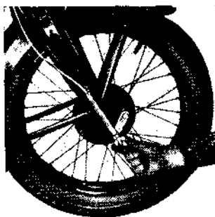
Abb. 17. Einstellen der Vorderradbremse. Das Nachstellen der Bremsen kann ohne jedes Werkzeug durch einfaches Rechtsdrehen des Knebels erreicht werden. Normalerweise genügen 2 Umdrehungen. Nach dem Einstellen ist zu prüfen, ob sich das Rad leicht drehen läßt (also die Bremsbacken voll öffnen!).
