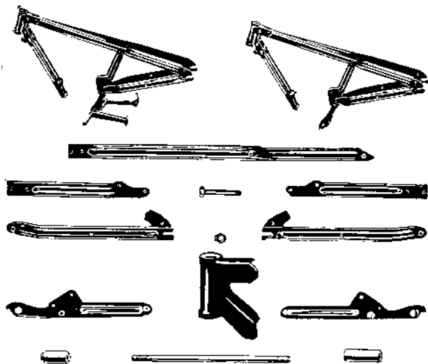
Abb. 37. Rahmen zerlegt.
