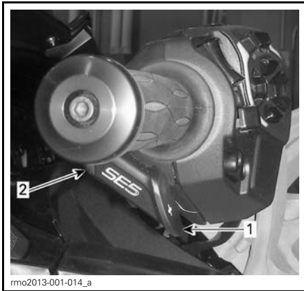
1. Upshift 2. Downshift
