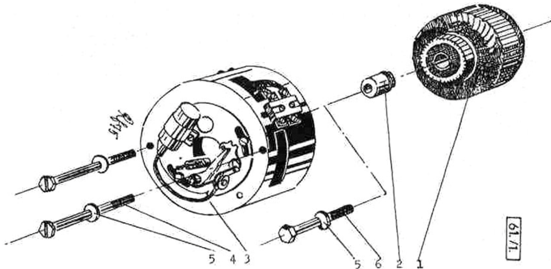
61/1. Generátor
