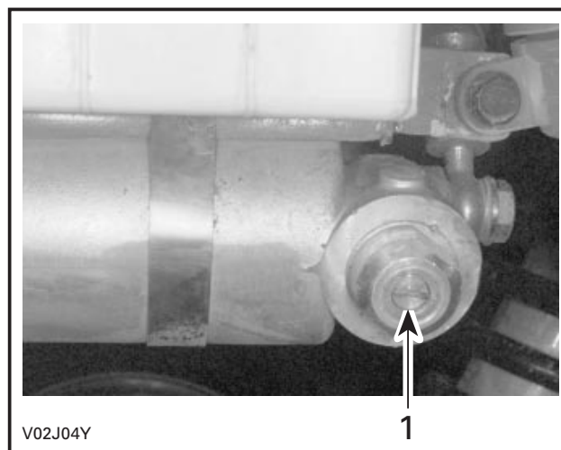
1. Adjuster
