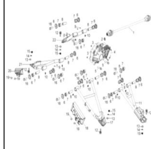
D-15: A-ARM
