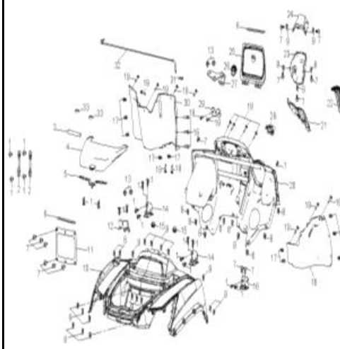
D-6: CAB
