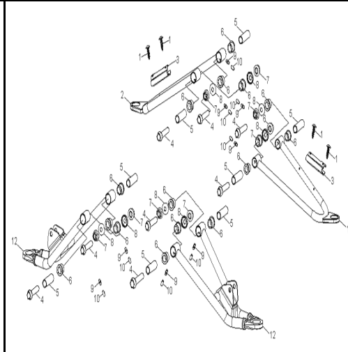
D-15: A-ARM
