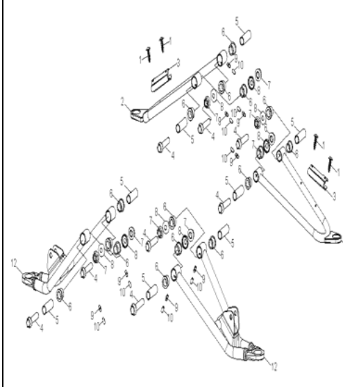
D-15: A-ARM
