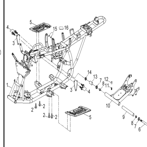
D-18: FRAME BODY
