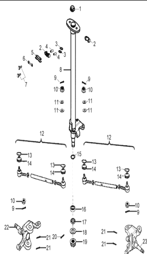
D-28: STEERING
