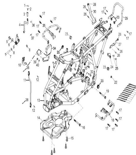
D-15: FRAME BODY
